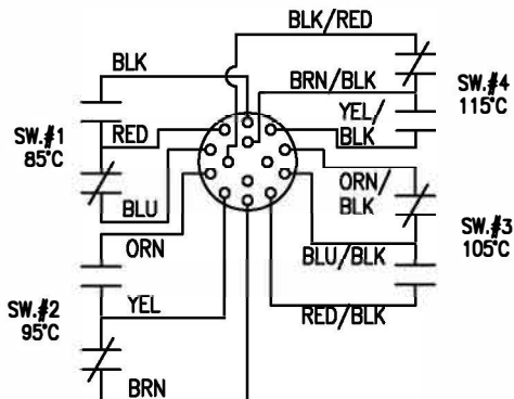
WIRING DIAGRAM-12A1
