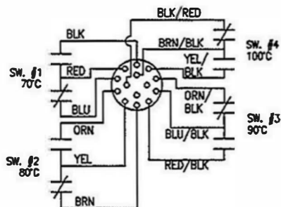
WIRING DIAGRAM-12A1
